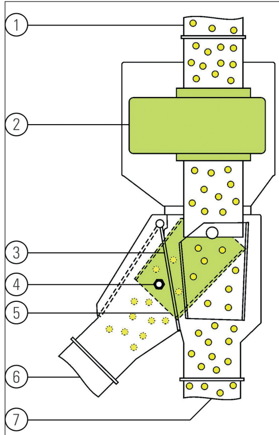
1) Inlet pipe 2) Detection coil 3) Sealing flap 4) Metal 5) Swivel hopper 6) Reject outlet 7) Material outlet
